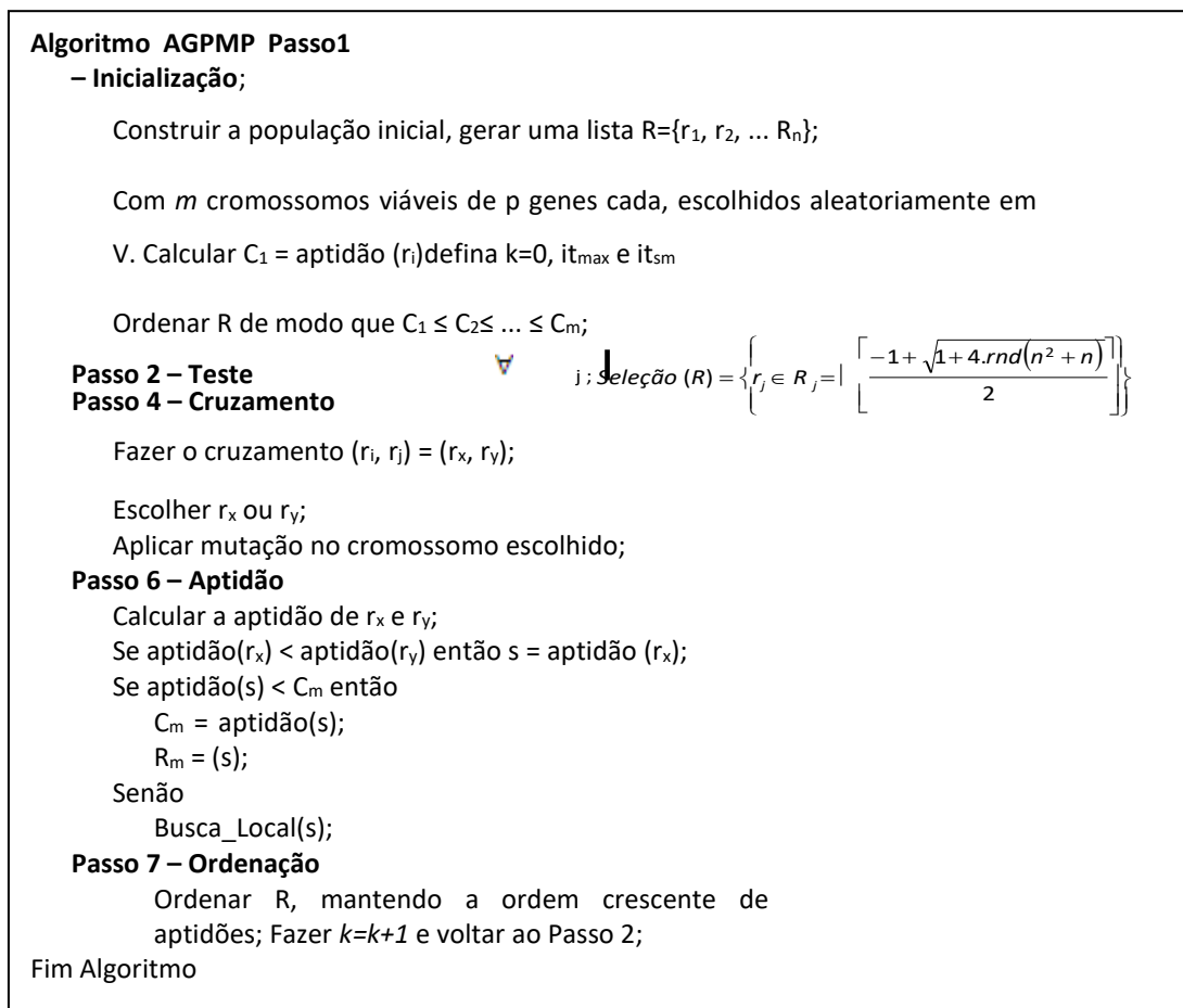
Figura 3 – Pseudocódigo do Algoritmo Genético para o PMP
