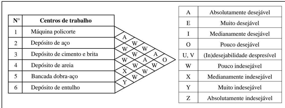
Figura 2: Classificação
