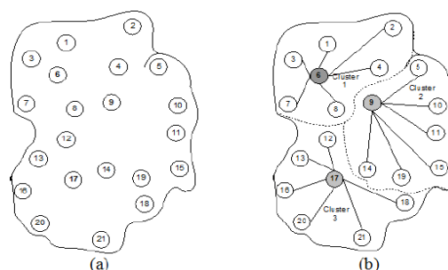
Figura 1 – p-Medianas
