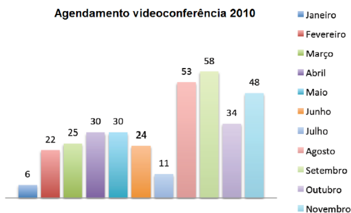
Gráfico 1– Agendamento videoconferência 2010
