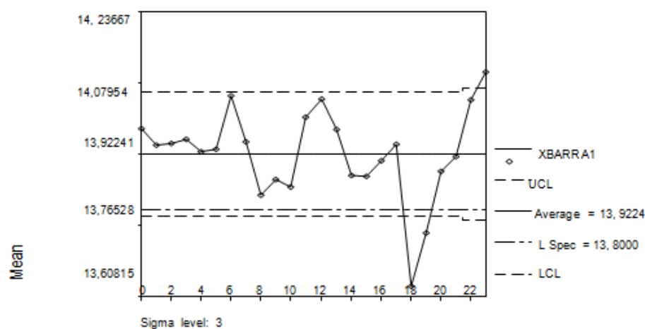
Figura 2: Gráfico de controle \bar{X} que representa o comportamento da tensão ao longo do dia para a subestação em análise
