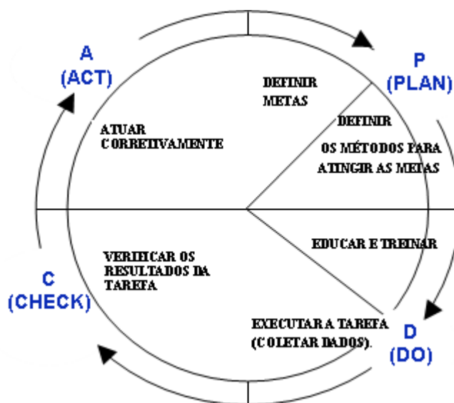
Figura 2 Ciclo PDCA
