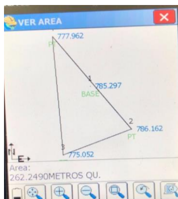
Figura 5 – Área calculado pelo GNSS Topográfico
